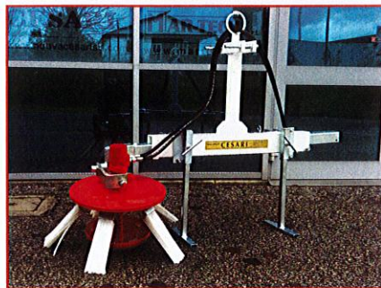
RAP1 al sollevatore anteriore o posteriore RAP1 to front or back lift
